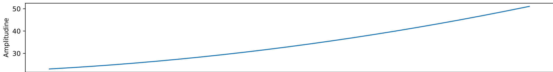
Trend
