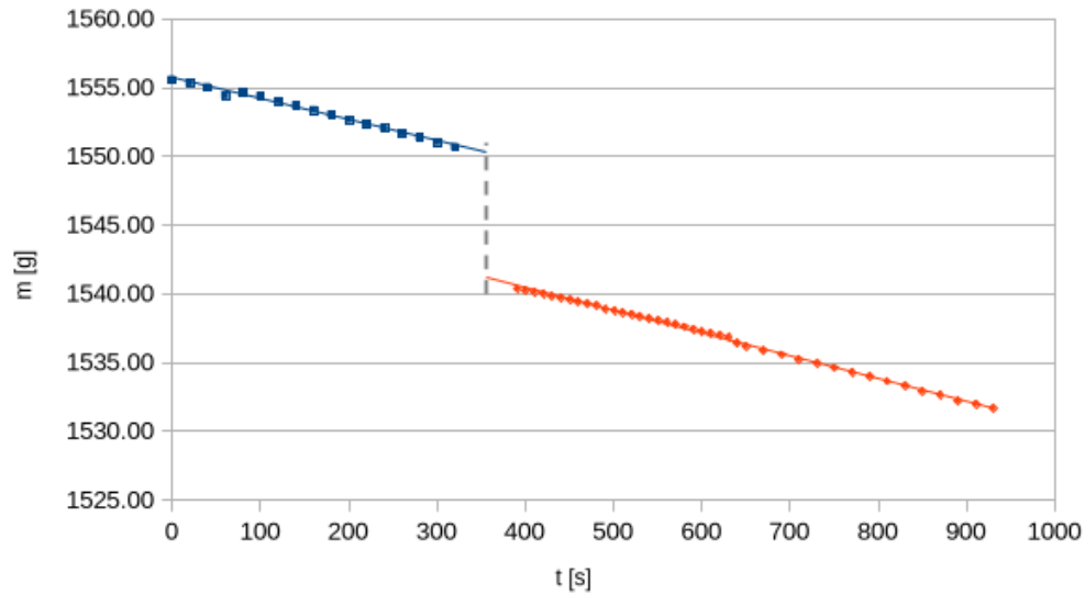
Figura 3: Andamento temporale della variazione di massa nel calorimetro. Le linee rette indicano i fit lineari di background estrapolati fino all'istante medio dell'immersione t_m = 355.575 \text{ s} .
