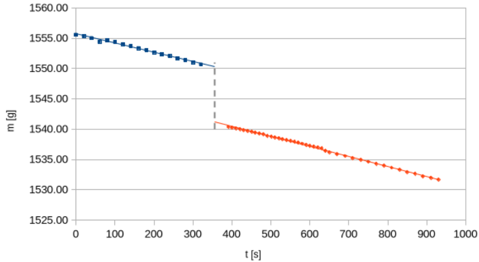
Figura 3: Andamento temporale della variazione di massa nel calorimetro. Le linee rette indicano i fit lineari di background estrapolati fino all'istante mediano dell'immersione t_m = 355.575 s.
