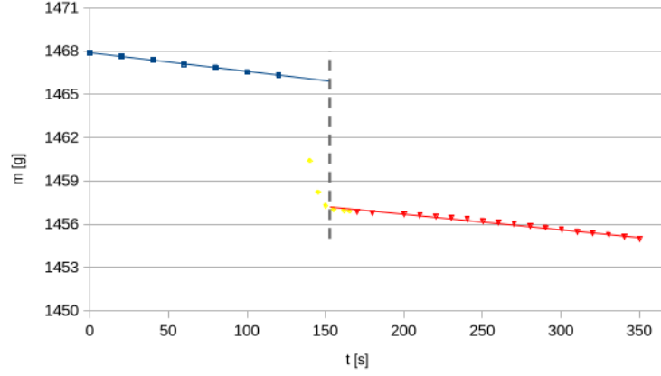
Figura 4: Andamento temporale della massa del secondo tentativo. Le linee indicano i fit di background estrapolati all'istante t_m = 152.7 s.
