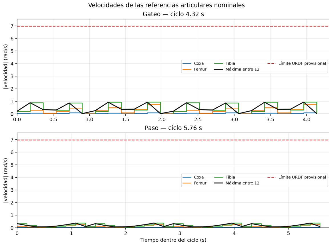
FIGURA 2: Envolturas de velocidad de coxa, fémur y tibia, y máximo entre las doce articulaciones, para las referencias nominales de gateo y paso. La línea discontinua indica el límite provisional del URDF.
