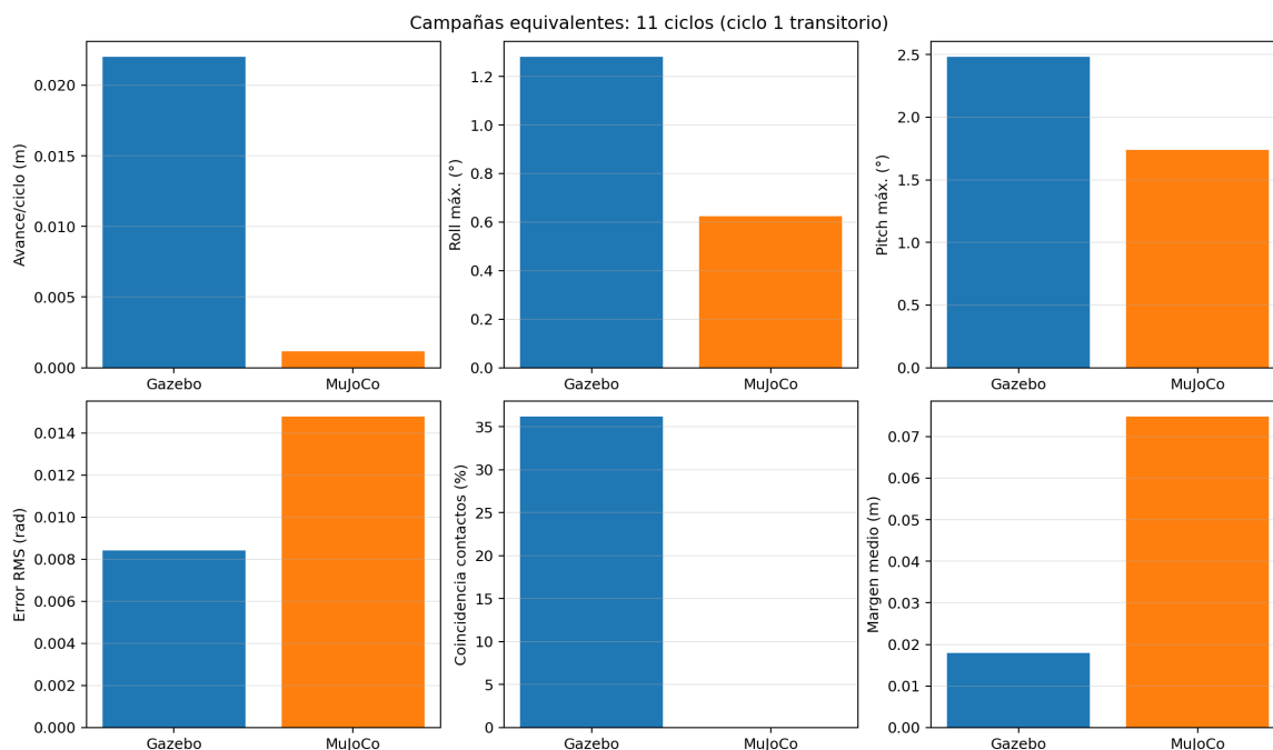
FIGURA 13: Comparación de avance, orientación, seguimiento, contactos y margen en 11 ciclos equivalentes de Gazebo y MuJoCo. La interfaz es común, pero las diferencias dinámicas permanecen sujetas a identificación física.
