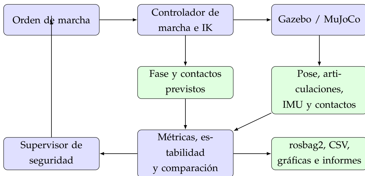
FIGURA 3: Arquitectura funcional implementada para generación, simulación, monitoreo, seguridad y registro de evidencia. Fuente: elaboración propia.
