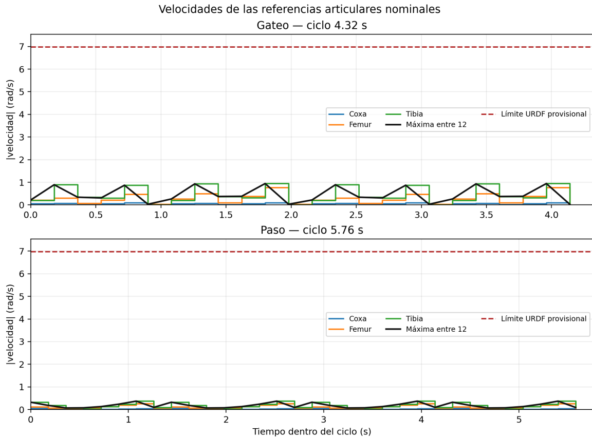
FIGURA 2: Envolventes de velocidad de coxa, fémur y tibia, y máximo entre las doce articulaciones, para las referencias nominales de gateo y paso. La línea discontinua indica el límite provisional del URDF.
