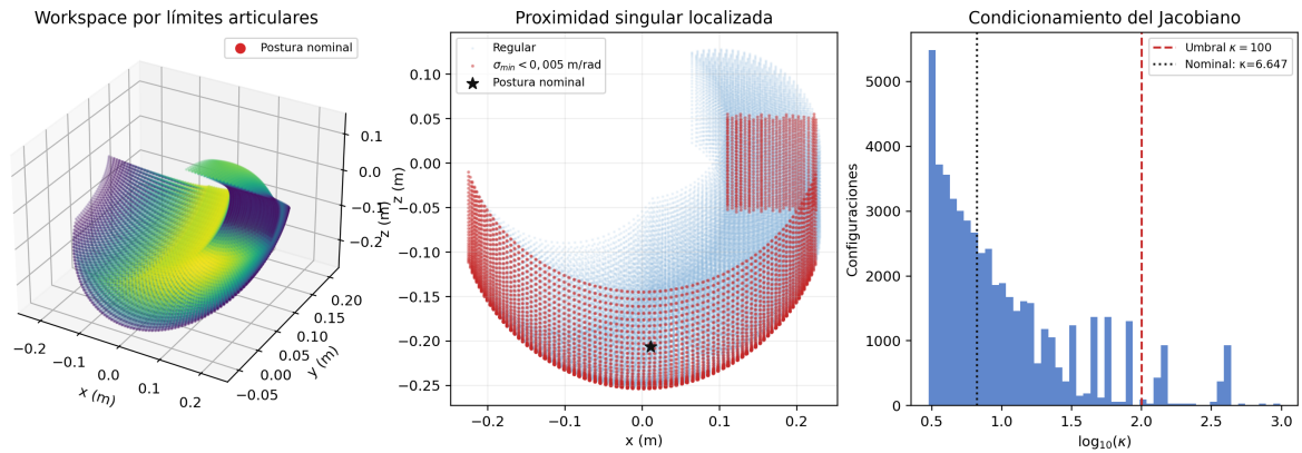
FIGURA 1: Workspace cinemático, localización de configuraciones próximas a singularidad y distribución del número de condición del Jacobiano para una pata izquierda. Fuente: elaboración propia.
