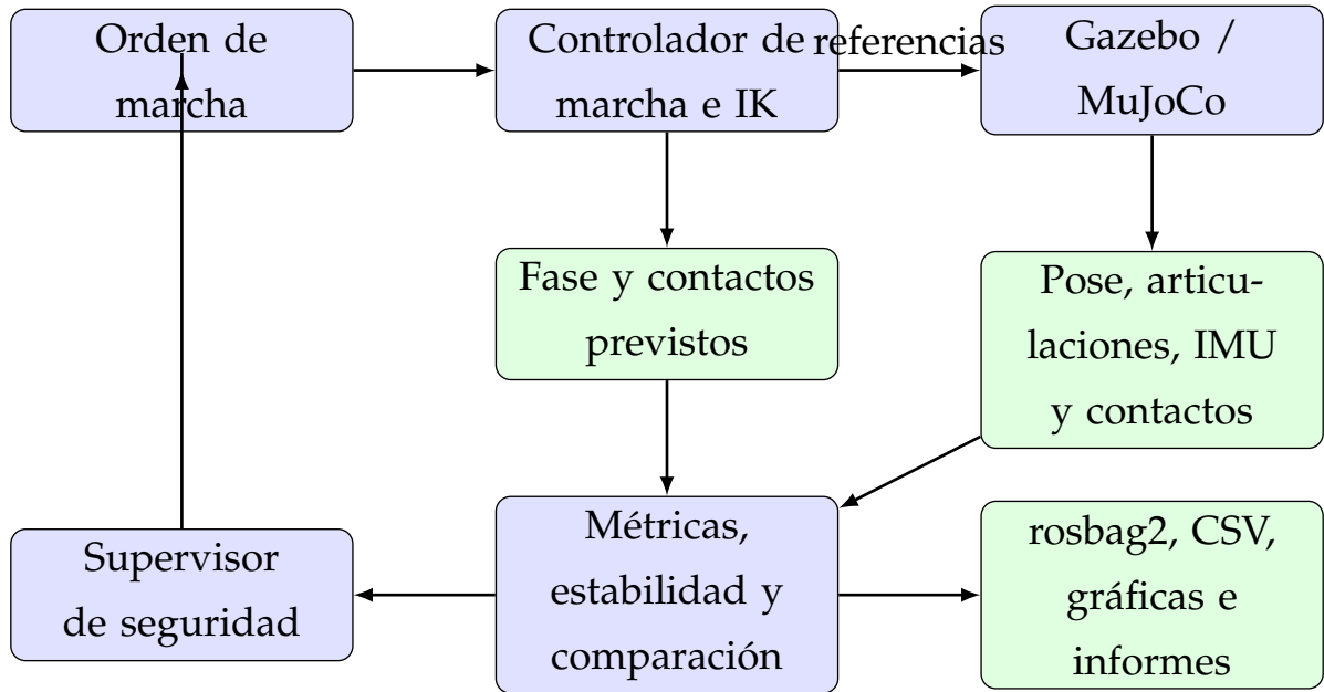
FIGURA 1: Arquitectura funcional implementada para generación, simulación, monitoreo, seguridad y registro de evidencia. Fuente: elaboración propia.
