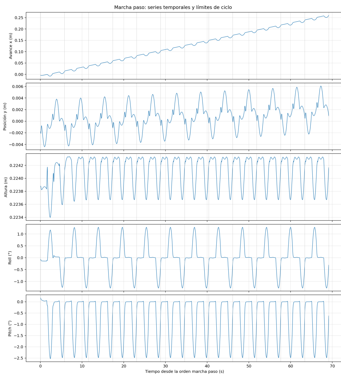
FIGURA 4: Series temporales de la línea base de marcha paso en Gazebo. Fuente: elaboración propia a partir de la bolsa paso_linea_base_20260814 .
