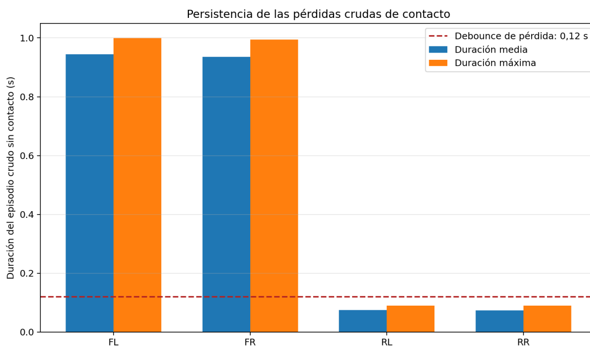
FIGURA 11: Duración media y máxima de los episodios crudos sin contacto. La línea discontinua representa la persistencia adicional exigida para confirmar una pérdida filtrada. Fuente: elaboración propia a partir de 24 ciclos del ensayo nominal válido del 1 de septiembre de 2026.
