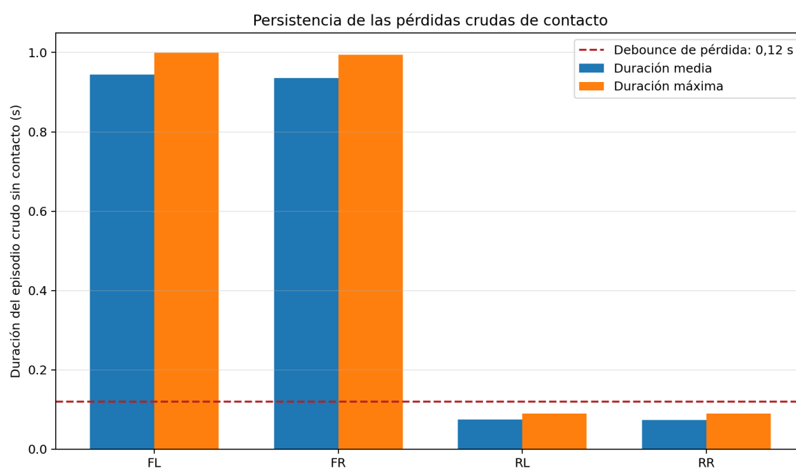
FIGURA 10: Duración media y máxima de los episodios crudos sin contacto. La línea discontinua representa la persistencia adicional exigida para confirmar una pérdida filtrada. Fuente: elaboración propia a partir de 24 ciclos del ensayo nominal válido del 1 de septiembre de 2026.
