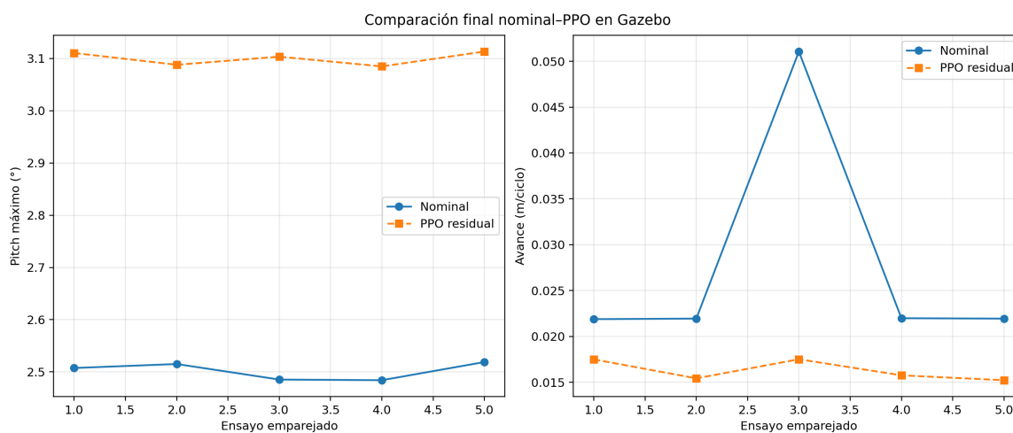
FIGURA 5: Comparación emparejada de cinco ensayos nominales y cinco ensayos con PPO residual en Gazebo.
