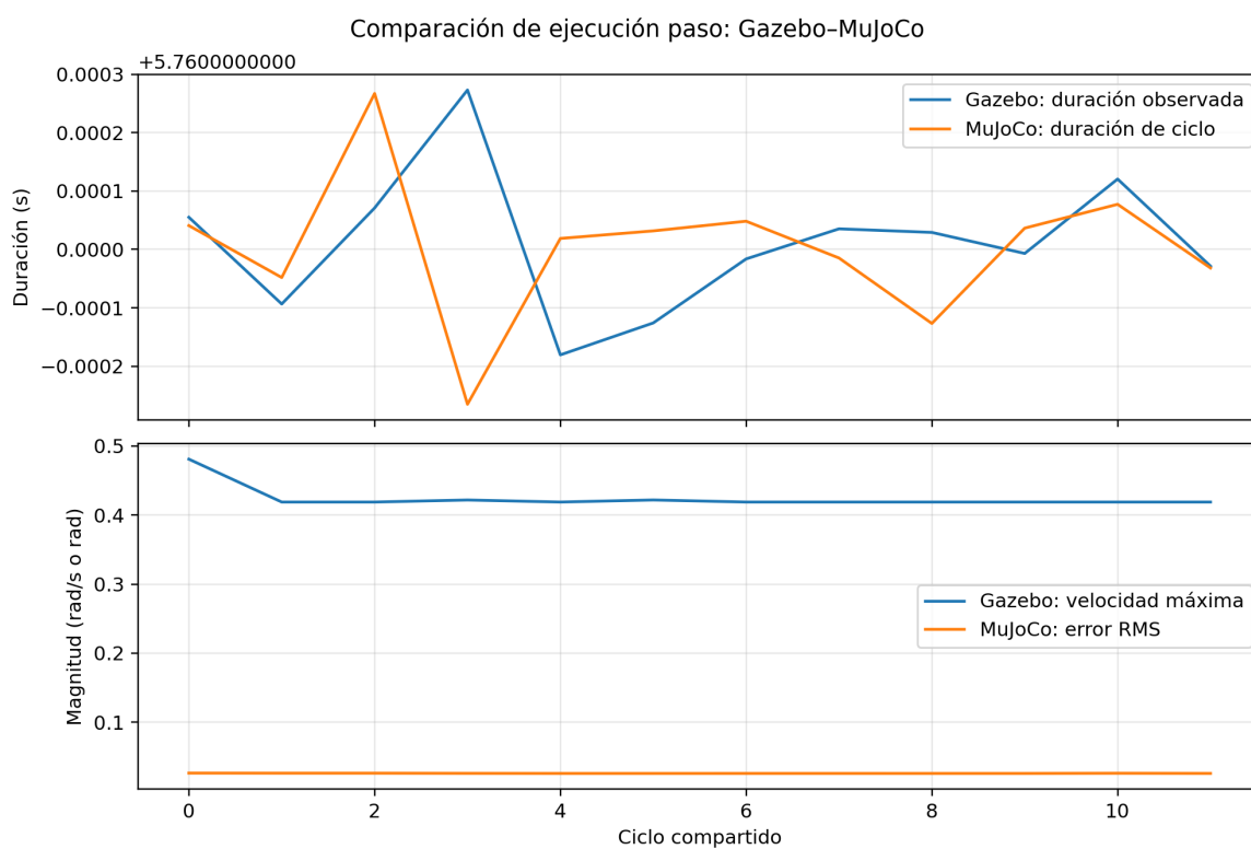
FIGURA 11: Comparación ciclo a ciclo de las magnitudes registradas en Gazebo y MuJoCo para la marcha paso. La equivalencia de contactos e IMU queda pendiente de una nueva bolsa MuJoCo con los sensores expuestos en ROS 2.
