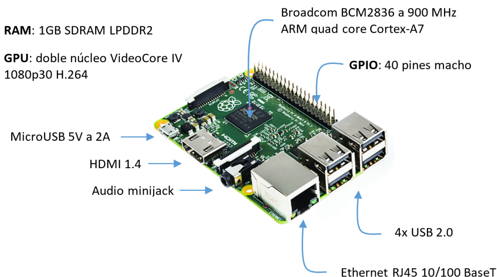
Figura 4.5: Especificaciones de Raspberry Pi 2B. Imagen de https://raspberryparatorpes.net modificada por mí[5].
