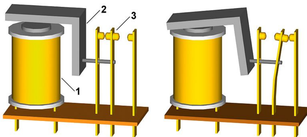
Figura 4.6: Estructura interna de un relé. Imagen de https://https://commons.wikimedia.org/[9]
