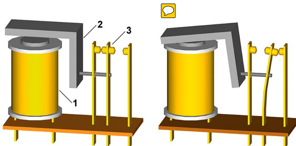
Figura 4.6: Estructura interna de un relé. Imagen de https://commons.wikimedia.org/[13]
