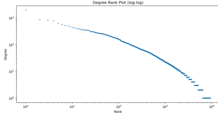
(d) Degree-Rank plot, network reale
