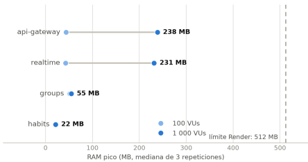
RAM pico por servicio: 100 → 1 000 VUs
