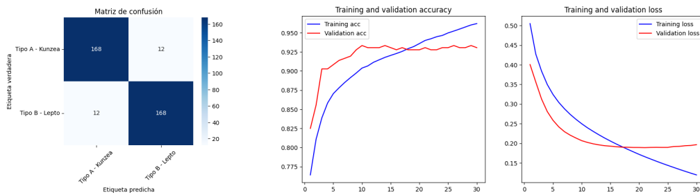
Figura 2: Matriz de confusión de una red densa con capas ocultas para el conjunto de testeo y la evolución de la función de pérdida en los conjuntos de entrenamiento y validación.
