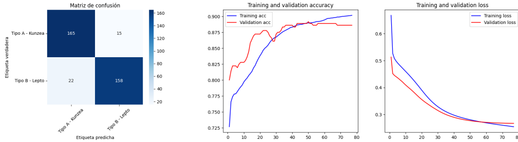
Figura 5: Matriz de confusión de la red 3 con regulación L2 para el conjunto de testeo y la evolución de la función de pérdida en los conjuntos de entrenamiento y validación.
