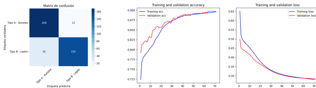
Figura 5: Matriz de confusión de la red 3 con regulación L2 para el conjunto de testeo y la evolución de la función de pérdida en los conjuntos de entrenamiento y validación.
