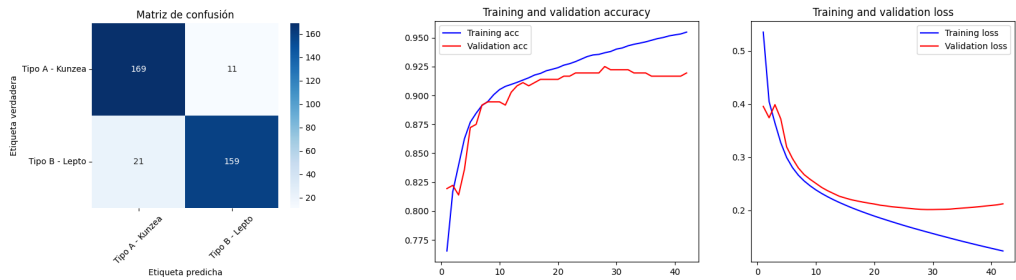
Figura 4: Matriz de confusión de la red 3 con una tercera capa convolucional para el conjunto de testeo y la evolución de la función de pérdida en los conjuntos de entrenamiento y validación.
