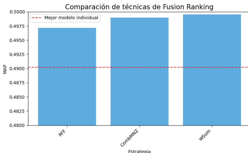
Figura 4.5: Comparativa de las técnicas de fusión evaluadas en términos de MAP con respecto al valor máximo individual alcanzado por los modelos.
