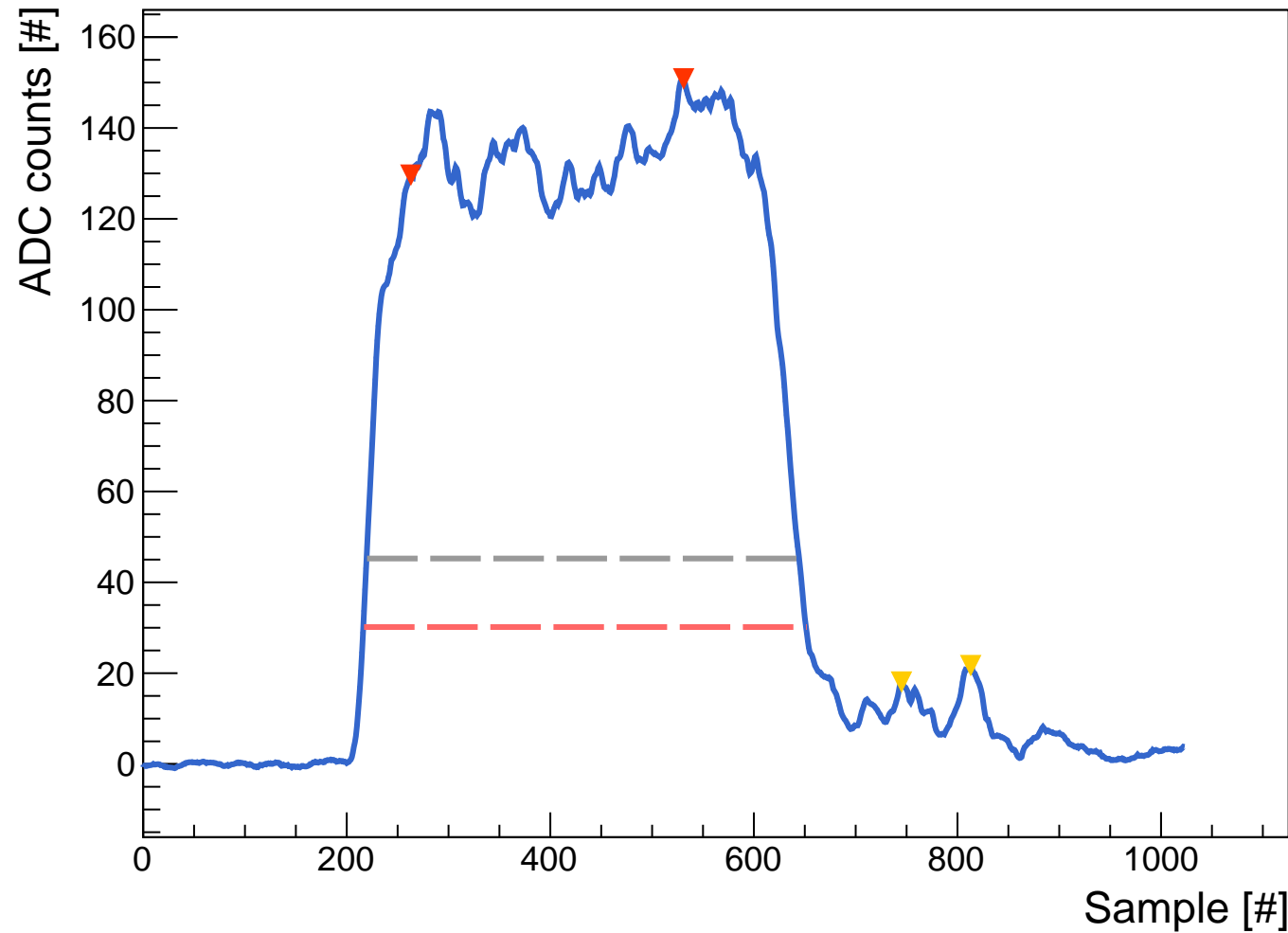
WF_run_41506_evt_276_trg_3_ch_2
