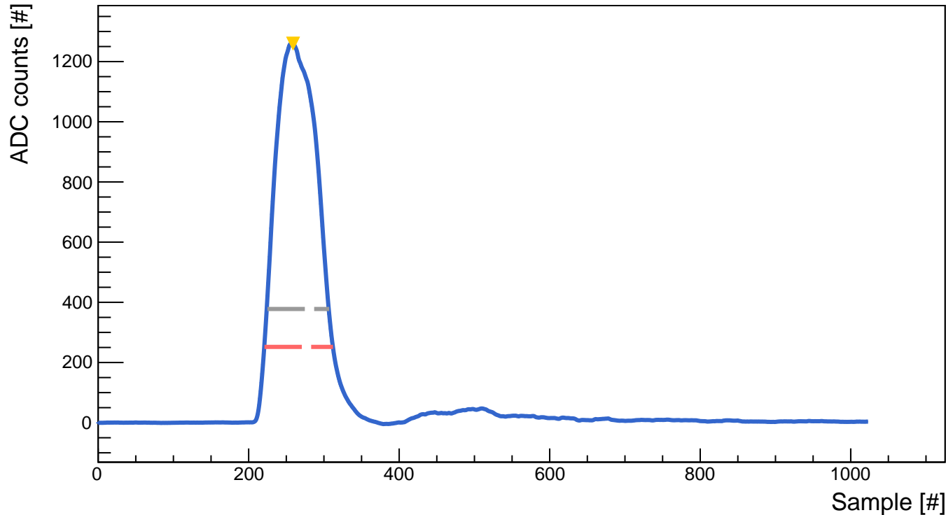
WFtest_run_22100_evt_89_trg_1_ch_1
