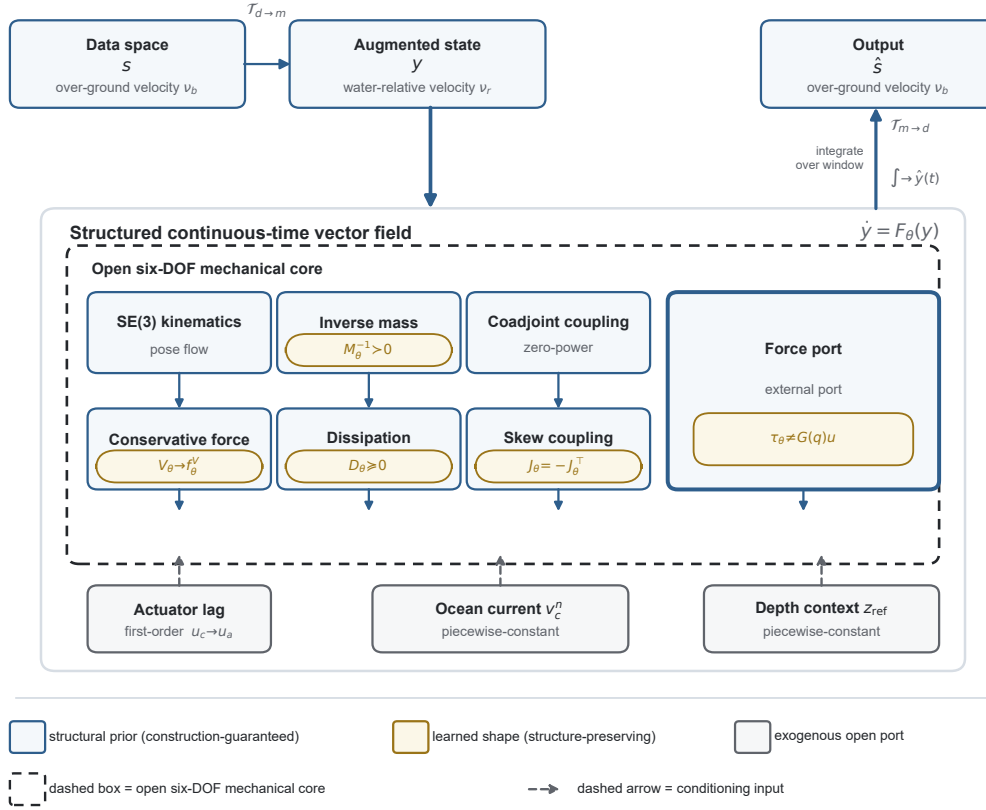
图 1.3: AUVHamNODE 核心方法与完整模型对象（本章主图）。数据态 s 经速度契约 \tau_{d \rightarrow m} （式 (1.26)）转换为增强模型态 y ，作为结构化连续时间向量场 \dot{y} = F_\theta(y) （式 (1.45)）的状态，在单个积分窗口内积分得 \hat{y}(t) ，再经 \tau_{m \rightarrow d} 映回数据空间得输出 \hat{s} 。配色区分三类语义：蓝色为参数化构造保证的结构先验，金色为保结构约束类内由网络学习的形状，灰色为外源开放端口；虚线框为开放式六自由度机械核心。各组件的结构约束、外源通道位置与适用边界见正文（第 1.5 节及第 1.6 节）；Fossen 功率角色到结构组件的转换见第 1.4 节，速度契约与机械核心功率关系分别见图 1.1 与图 1.4。
