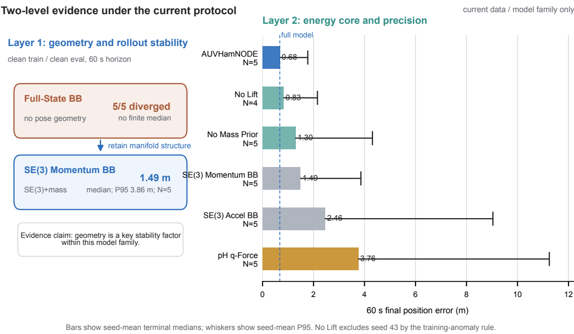
图 1.3: 当前证据集下的两级结构证据。左侧概括几何层证据：在干净初值训练和干净评估配置下，全状态黑箱五个随机种子全部长期递推发散，而保留 SE(3) 位姿运动学与常质量结构的动量黑箱保持有限误差。右侧概括能量与消融层证据：条形为 60 s 终端位置误差中位数的种子间均值，细线为 P95 的种子间均值。无升力耦合消融按统一训练异常判据排除随机种子 43；全状态黑箱因全部随机种子递推发散，不报告有限中位数。该图仅概括当前数据协议与模型族下的证据，不构成普遍必要性定理。
