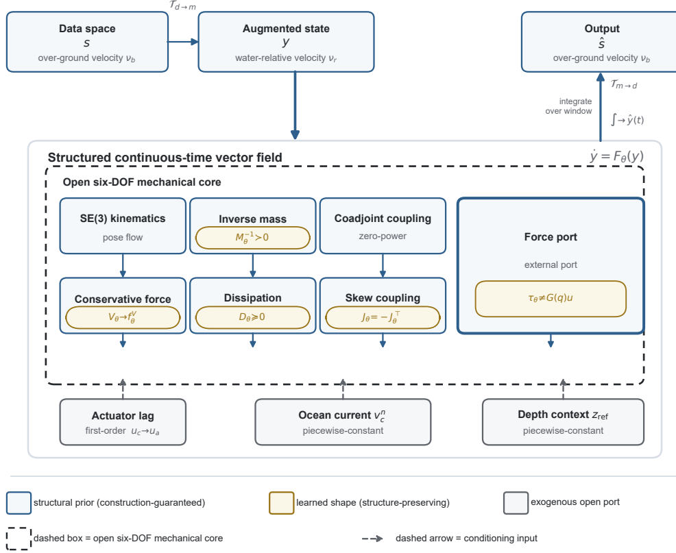
图 1.3: AUVHamNODE 核心方法与完整模型对象（本章主图）。数据态 s 经速度契约 \mathcal{T}_{d \rightarrow m} （式 (1.26)）转换为增强模型态 y ，并在结构化连续时间向量场 \dot{y} = F_\theta(y) （式 (1.45)）中积分得到 \hat{y}(t) ，再经 \mathcal{T}_{m \rightarrow d} 映回数据空间，得到输出 \hat{s} 。配色区分三类语义：蓝色表示参数化构造保证的结构先验，金色表示结构保持约束类内由网络学习的形状，灰色表示外源开放端口；虚线框表示开放式六自由度机械核心。各组件的结构约束、外源通道位置与适用边界见第 1.5 节和第 1.6 节；Fossen 功率角色到结构组件的转换见第 1.4 节，速度契约与机械核心功率关系分别见图 1.1 和图 1.4。
