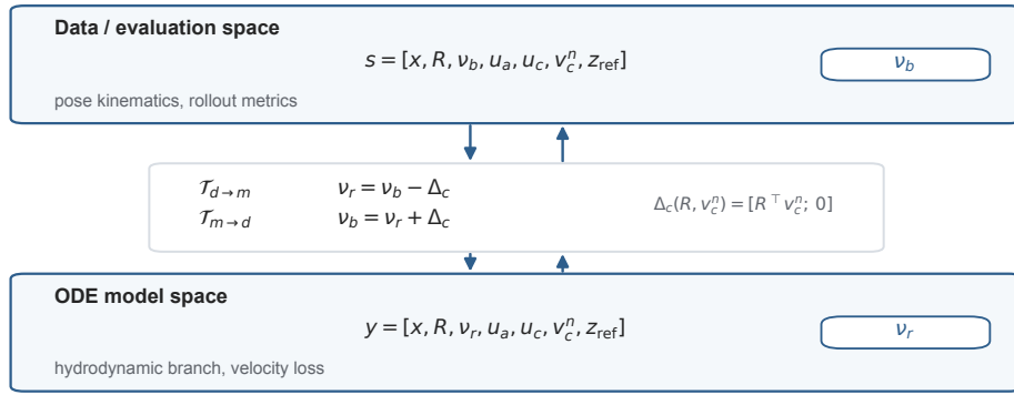
图 1.1: 海流条件下, 数据与评估空间和 ODE 模型空间之间的速度表示转换。数据与评估空间保留总体速度, ODE 模型空间使用相对水速度; 训练中的速度监督在模型空间进行, 输出报告和外部任务评估前再恢复总体速度。
