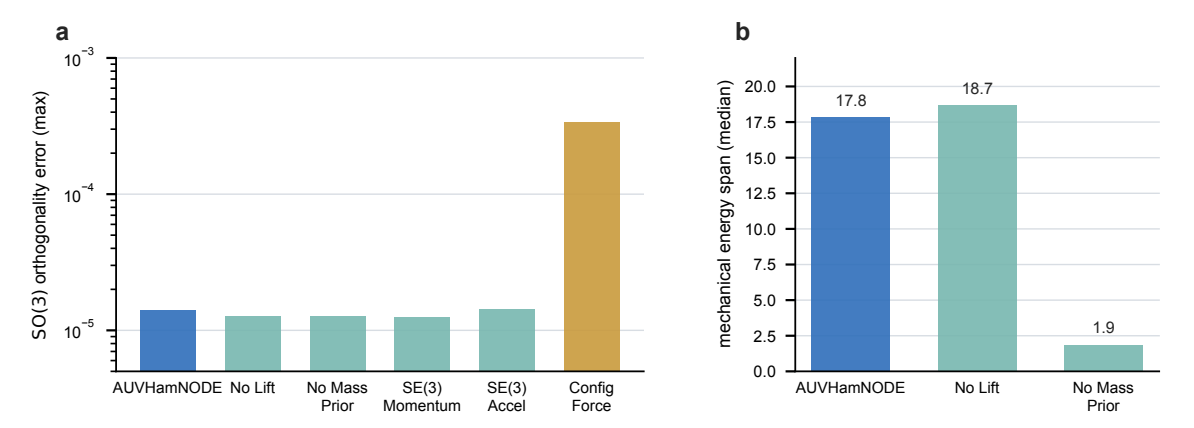
图 1.11: 干净配置下的内部结构诊断 (60 s 自由演化)。(a) 各模型 SO(3) 正交性误差最大值：保留 SE(3) 参数化的模型均在 1.3 \times 10^{-5} 量级，配置广义力基线约 3.4 \times 10^{-4} 、高约一个量级。(b) 机械能量跨度中位数：仅含标量势能核心的模型有定义（完整模型、无升力耦合与无质量先验消融），移除标量势能或不含能量语义的模型该量无定义、未列入。全状态黑箱因长期发散未纳入诊断。
