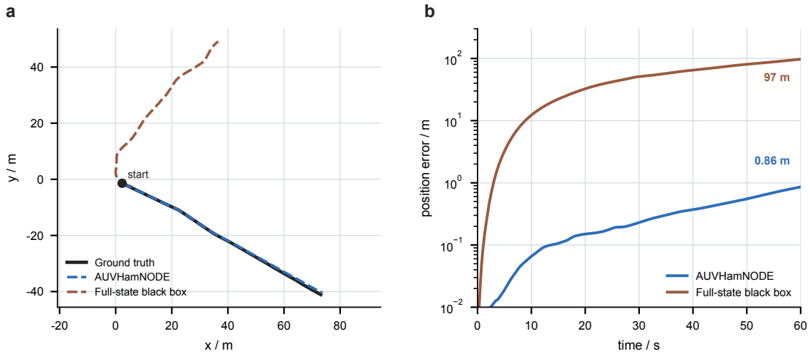
图 1.7: 一条多正弦扫频评估轨迹上完整模型与全状态黑箱的 60 s 自由演化对照。(a) 水平面俯视轨迹: 完整模型预测与真值几乎重合, 全状态黑箱的预测轨迹迅速偏离真值。(b) 位置误差随时间的增长 (对数纵轴): 完整模型终端误差约 0.86 m, 全状态黑箱累积至约 97 m。该轨迹为定性示例。
