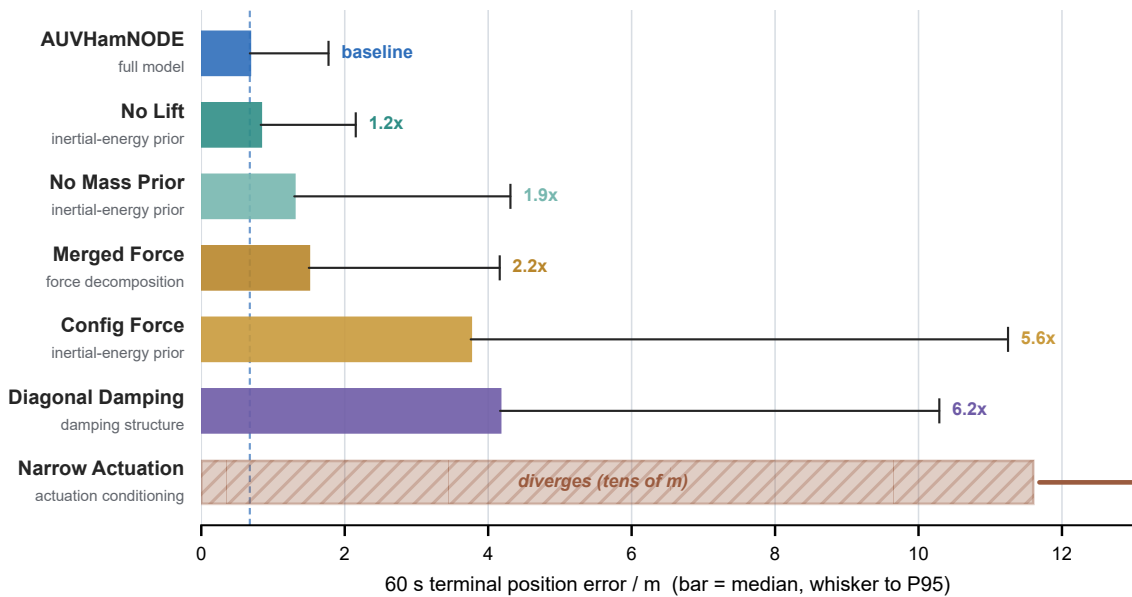
图 1.8: 结构成分逐项移除或改组的精度阶梯。条形表示 60 s 终端位置误差中位数，须线延伸至 P95；竖虚线表示完整模型基线，标注的倍数均相对于该基线计算。各行按所属结构轴标注，包括惯性-能量先验、耗散结构、广义力组织和广义力条件化。对角阻尼消融的终端误差中位数约为 4.2 m（六次重复），合并广义力基线约为 1.5 m（三次重复）。广义力条件化消融的六次重复全部长期发散，终端误差达到数十米量级，按长期稳定性失败处理，不计入有限阶梯；全状态黑箱因同样长期发散，也未列入。
