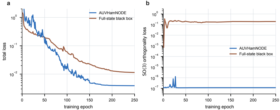
图 1.5: 干净初值训练下的训练动力学（曲线为重复训练间逐 epoch 中位数）。（a）训练总损失：结构化模型与全状态黑箱均稳定收敛，黑箱收敛到略高的损失水平。（b）SO(3) 正交性损失：结构化模型将其压至 10^{-7} 量级，全状态黑箱则全程维持在约 0.2 量级的高位；该量独立于任务损失，预示黑箱在长期自由演化中的姿态发散。
