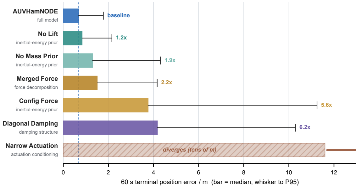
图 1.8: 结构成分逐项移除或改组后的精度比较。条形表示 60 s 终端位置误差中位数，须线延伸至 P95；竖虚线表示完整模型基线，标注的倍数均相对于该基线计算。各行按结构因素分组，包括惯性与能量相关先验、耗散结构、广义力组织方式和广义力分支输入变量。对角阻尼消融的终端误差中位数约为 4.2 m（六次重复），合并广义力基线约为 1.5 m（三次重复）。广义力分支输入消融的六次重复全部长期发散，终端误差达到数十米量级，按长期稳定性失败处理，不计入有限值比较；全状态黑箱因同样长期发散，也未列入。
