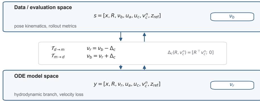
图 1.1: 海流条件下，数据与评估空间和 ODE 模型空间之间的速度表示转换。数据与评估空间保留绝对广义速度，ODE 模型空间使用相对水体广义速度；训练中的速度监督在模型空间进行，输出报告和外部任务评估前再恢复绝对广义速度。
