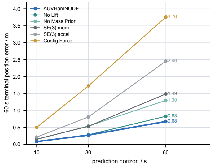
图 1.6: 表 1.11 中各有限模型 60 s 自由演化终端位置误差中位数随评估时域 (10、30、60 s) 的增长 (重复训练间均值)。结构化模型与半结构化黑箱误差随时域平滑增长并保持有限; 全状态黑箱因全部重复长期发散、无有限曲线, 故未列入。
