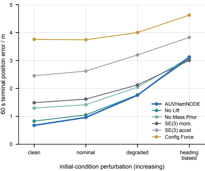
图 1.10: 干净初值训练下终端位置误差中位数随评估端初值扰动配置（干净、名义、退化、航向偏置）的变化（重复训练间均值）。横轴前三档为随机强度递增序列，航向偏置为叠加固定偏航偏置的系统性误差档，各档按其诱发的终端误差从小到大排列。完整模型的精度领先随扰动增强逐步收窄，在诱发误差最大的航向偏置评估下与若干结构化基线及 SE(3) 动量黑箱相互收敛；全状态黑箱在所有扰动配置下均长期发散、无有限曲线。
