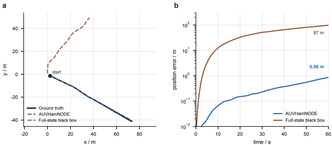
图 1.7: 一条多正弦扫频评估轨迹上完整模型与全状态黑箱的 60 s 自由演化对照。(a) 水平面俯视轨迹: 完整模型预测与真值几乎重合, 全状态黑箱预测偏离真值。(b) 位置误差随时间的增长 (对数纵轴): 完整模型终端误差约 0.86 m, 全状态黑箱累积至约 97 m。该轨迹为定性示例。
