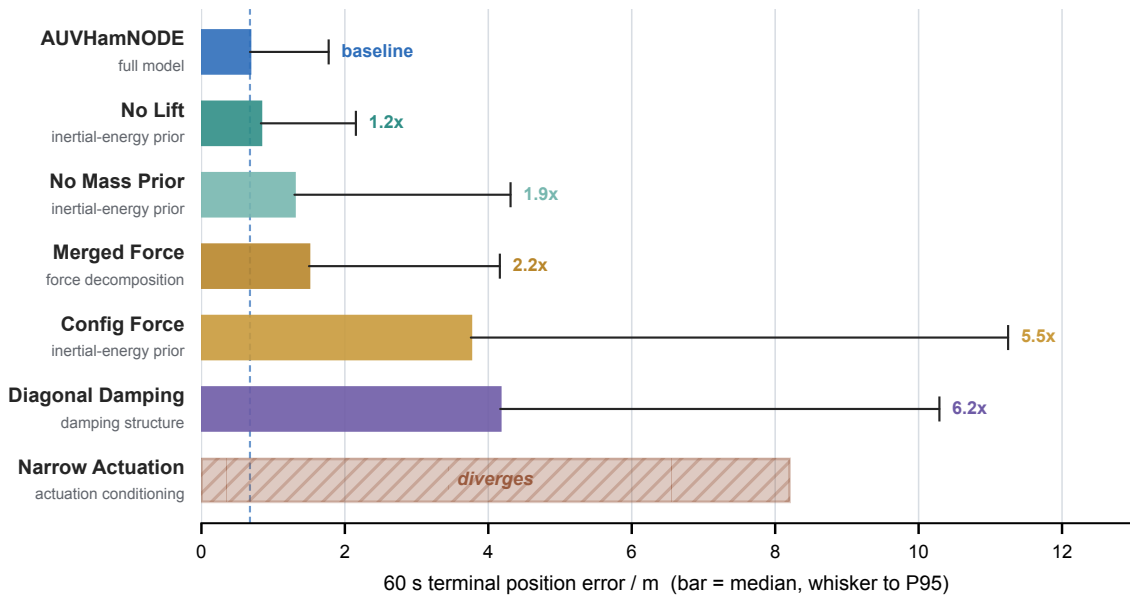
图 1.8: 结构成分逐项移除或改组的精度阶梯。条形为 60 s 终端位置误差中位数、须线延伸至 P95, 竖虚线为完整模型基线, 标注的倍数均相对该基线计; 各行按其所属结构轴标注 (惯性-能量子先验、耗散结构、广义力组织、广义力条件化)。对角阻尼消融的终端误差中位数约 4.2 m (六次重复), 合并广义力基线约 1.5 m (三次重复)。广义力条件化消融的六次重复全部长期发散、终端误差达数十米量级, 按长期稳定性失败处理、不计入有限阶梯; 全状态黑箱因同样长期发散亦未列入。
