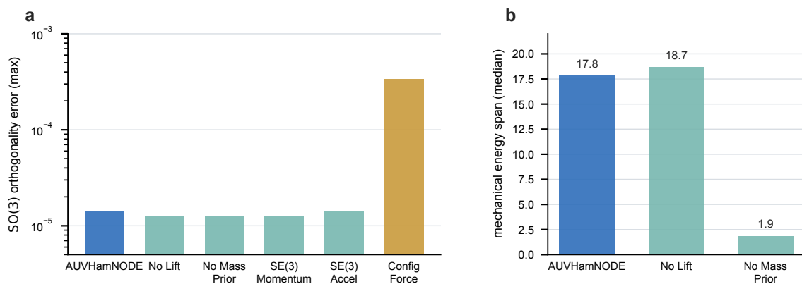
图 1.11: 干净配置下的内部结构诊断 (60 s 自由演化)。(a) 各模型 SO(3) 正交性误差最大值: 保留 SE(3) 参数化的模型均在 1.3 \times 10^{-5} 量级, 配置广义力基线约 3.4 \times 10^{-4} 、高约一个量级。(b) 机械能量跨度中位数: 仅含标量势能核心的模型有定义 (完整模型、无升力耦合与无质量先验消融), 移除标量势能或不合能量语义的模型该量无定义、未列入。全状态黑箱因长期发散未纳入诊断。
