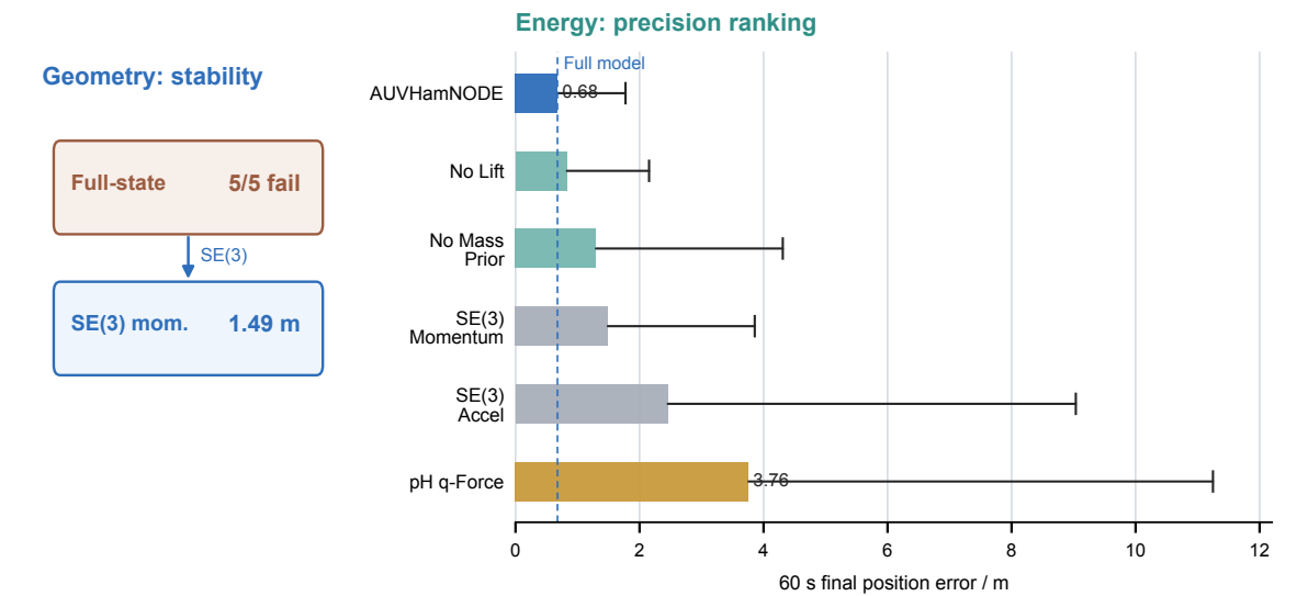
图 1.4: 当前证据集下的两级结构证据。左侧只概括几何层对照：全状态黑箱在五个随机种子上均长期递推发散，而保留 SE(3) 位姿运动学与常质量结构的动量黑箱保持有限误差。右侧给出能量与消融层的精度排序：条形为 60 s 终端位置误差中位数的种子间均值，细线为 P95 的种子间均值。无升力耦合消融按统一训练异常判据排除随机种子 43；全状态黑箱因全部随机种子递推发散，不报告有限中位数。该图仅概括当前数据协议与模型族下的证据，不构成普遍必要性定理。
