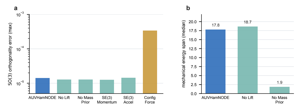
图 1.11: 干净配置下的内部结构诊断（60 s 自由演化）。(a) 各模型 SO(3) 正交性误差最大值：保留 SE(3) 参数化的模型均在 1.3 \times 10^{-5} 量级，配置广义力基线约 3.4 \times 10^{-4} 、高约一个量级。(b) 机械能量跨度中位数：仅含标量势能核心的模型有定义（完整模型、无升力耦合与无质量先验消融），移除标量势能或不含能量语义的模型该量无定义、未列入。全状态黑箱因长期发散未纳入诊断。
