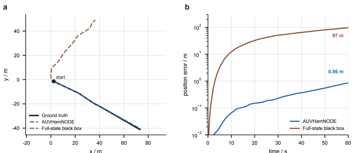
图 1.7: 一条多正弦扫频评估轨迹上完整模型与全状态黑箱的 60 s 自由演化对照。(a) 水平面俯视轨迹: 完整模型预测与真值几乎重合, 全状态黑箱预测窜离真值。(b) 位置误差随时间的增长 (对数纵轴): 完整模型终端误差约 0.86 m, 全状态黑箱累积至约 97 m。该轨迹为定性示例。
