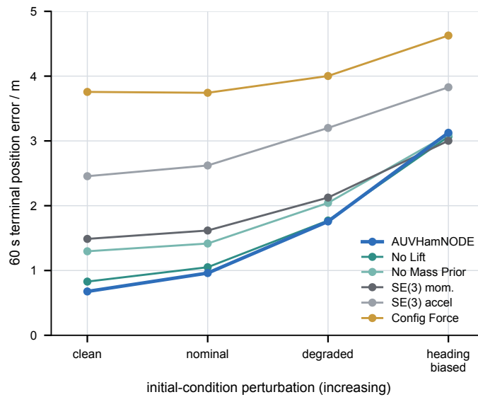
图 1.10: 干净初值训练下终端位置误差中位数随评估端初值扰动强度（干净、名义、退化、航向偏置）的变化（重复训练间均值）。完整模型的精度领先随扰动增强逐步收窄，在最强的航向偏置评估下与若干结构化基线及 SE(3) 动量黑箱相互收敛；全状态黑箱在所有扰动配置下均长期发散、无有限曲线。
