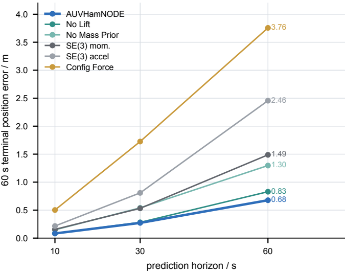
图 1.6: 各有限模型 60 s 自由演化终端位置误差中位数随评估时域（10、30、60 s）的增长（重复训练间均值）。结构化模型与半结构化黑箱误差随时域平滑增长并保持有限；全状态黑箱因全部重复长期发散、无有限曲线，故未列入。
