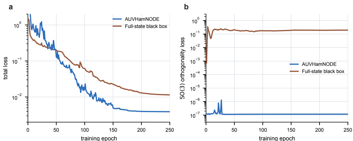
图 1.5: 干净初值训练下的训练动力学（曲线为重复训练间逐 epoch 中位数）。(a) 训练总损失：结构化模型与全状态黑箱均稳定收敛，黑箱收敛到略高的损失水平。(b) SO(3) 正交性损失：结构化模型将其压至 10^{-7} 量级，全状态黑箱则全程滞留在约 0.17 的高位；该量独立于任务损失之外，预示黑箱在长期自由演化中的姿态发散。
