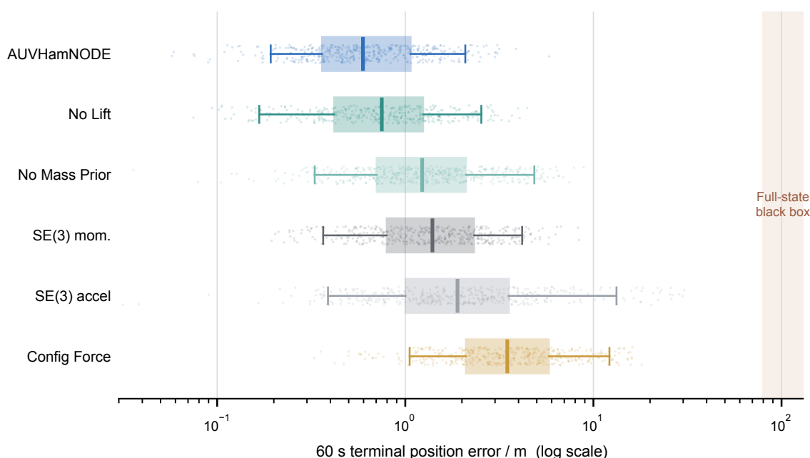
图 1.9: 各有限模型逐轨迹 60 s 终端位置误差分布（对数横轴；箱体为四分位距，须线为 P5–P95，箱内竖线为中位数）。无质量先验消融的中位数低于 SE(3) 动量黑箱，但其上尾更重，二者在中位数与 P95 上排序翻转。全状态黑箱因长期发散落在 80–90 m 量级（右侧阴影带），不参与有限分布比较。
