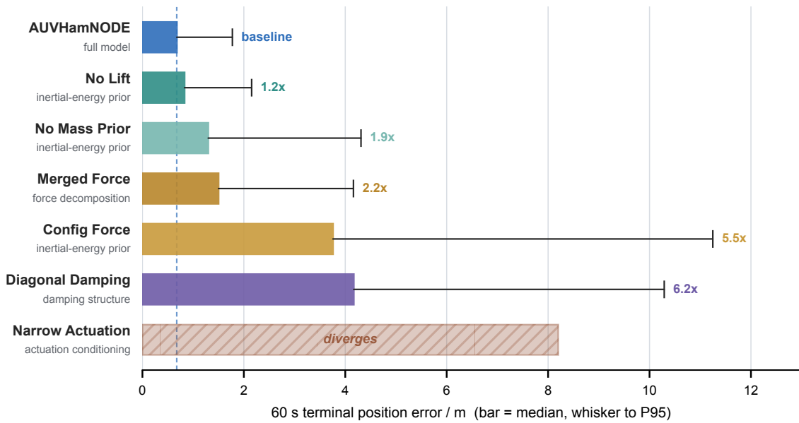
图 1.8: 结构成分逐项移除或改组的精度阶梯。条形为 60 s 终端位置误差中位数、须线延伸至 P95，竖虚线为完整模型基线，标注的倍数均相对该基线计；各行按其所属结构轴标注（惯性-能量子先验、耗散结构、广义力组织、广义力条件化）。广义力条件化消融全部重复长期发散，按长期稳定性失败处理、不计入有限阶梯；全状态黑箱因同样长期发散亦未列入。
