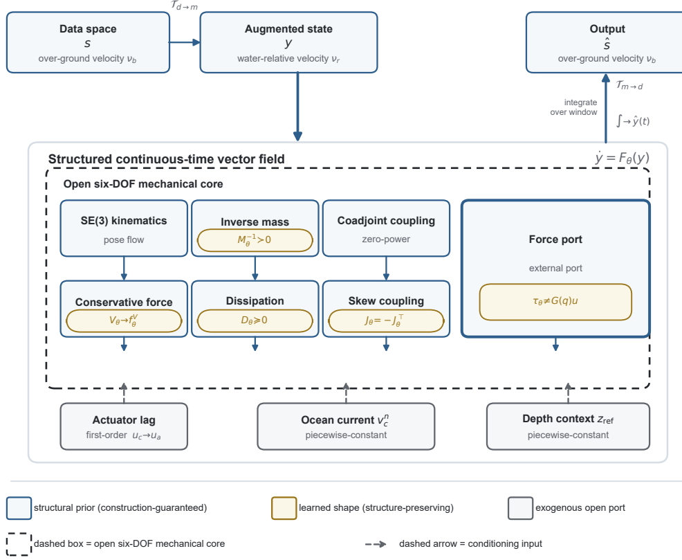
图 1.3: AUVHamNODE 方法与完整模型对象（本章主图）。数据态 s 经速度表示转换 T_{d \rightarrow m} （式 (1.26)）转换为增强模型态 y ，并在结构化连续时间向量场 \dot{y} = F_\theta(y) （式 (1.45)）中积分得到 \hat{y}(t) ，再经 T_{m \rightarrow d} 映回数据空间，得到输出 \hat{s} 。配色区分三类对象：蓝色表示参数化构造保证的结构先验，金色表示结构保持函数类内由网络学习的函数，灰色表示外源变量和外部广义力；虚线框表示开放式六自由度机械子系统。各组件的结构约束、外源变量位置与适用边界见第 1.5 节和第 1.6 节；Fossen 型动力学项与结构组件的对应关系见第 1.4 节，速度约定与该子系统的功率关系分别见图 1.1 和图 1.4。
