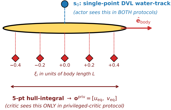
图 1: 任务与 sensor 协议示意。(a) D2Q9 TRT-LBM 离线生成的 Kármán 涡街尾迹场 ( U_\infty = 1.0 \text{ m/s} , \text{Re} = 150 , \text{Ti} = 5\% ) 的一帧涡量场背景, 叠加 REMUS-100 体示意 (黄色椭圆, 红色箭头为体轴朝向) 与 cross-stream 任务目标 (绿色五角星)。(b) 体坐标系下两种 sensor 抽样协议: 蓝色实心圆 s_0 是部署可获得的单点 DVL 水追踪 (actor 在两种协议下都只读这一通道); 红色菱形为 \xi_i \in \{-0.4, -0.2, 0, +0.2, +0.4\} \cdot L 沿体轴的 5 个等距采样点, 等权平均后给出壳积分等效水流 \mathbf{o}^{\text{priv}} = [u_{\text{eq}}, v_{\text{eq}}] ——仅在 privileged-critic protocol 训练阶段被 critic 读取, 部署阶段不可用 ((2))。
