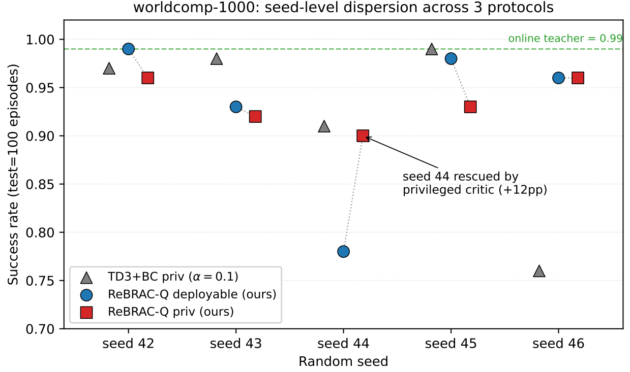
图 2: seed-level success rate 分布 (worldcomp-1000, test=100 episodes) 。横轴为 5 个 random seeds (42–46)，纵轴为成功率。三种协议：(i) TD3+BC privileged-critic ( \alpha = 0.1 , 灰色三角)；(ii) ReBRAC-Q deployable-only (蓝色圆点)；(iii) ReBRAC-Q privileged-critic (红色方块)。同一 seed 之间用细虚线连接，便于读出“deployable→privileged”在 seed 内部的位移。 关键观察 ：seed 44 在 ReBRAC-Q deployable-only 下显著低于其他 seed (0.78 vs 0.93–0.99)，切换到 privileged-critic 后被救回到 0.90 (+12pp)；其他 seed 的“deployable→privileged”位移均在 \pm 3\text{pp} 内，方向并不一致——privileged-critic 在 ReBRAC-Q 上的 mean 抬升完全由 seed 44 这一个 outlier 提供。
