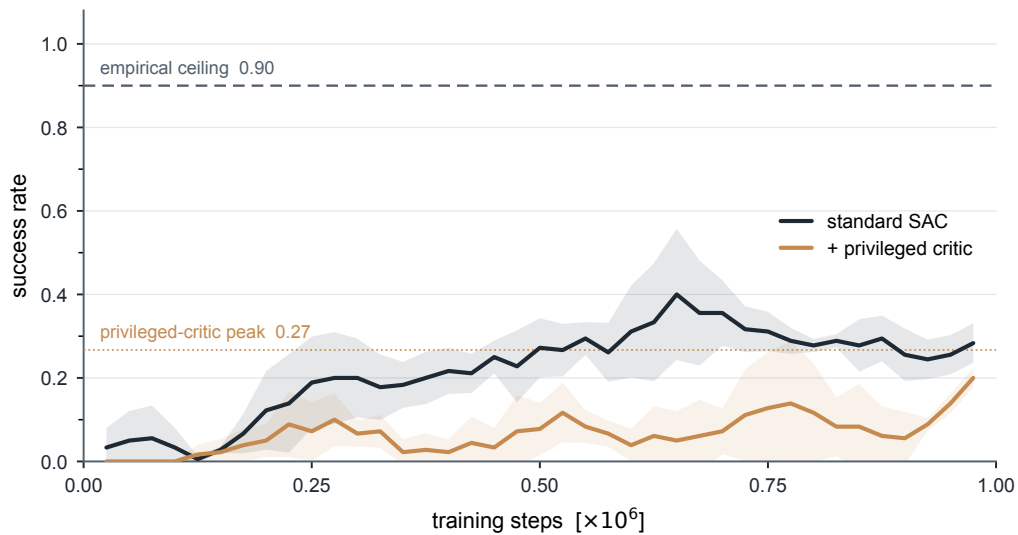
图 5.7: 反向对照: 临界工况下向价值网络注入特权来流观测对可部署成功率的作用 (学习曲线, 均值与种子带, 曲线经轻度滑动平均)。自同一 k = 4 基线, 注入特权观测后成功率在整个训练过程中低于标准 SAC, 其峰值跨重复训练稳定锁定在约 0.27 (暖色点线) 而不能逾越——与延长时序窗的方向相反。可部署性能的瓶颈在策略对单点观测的时序利用, 而非价值一侧的信息或估计能力。
