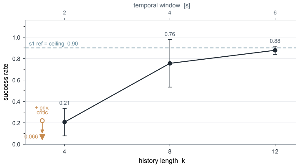
图 5.5: 临界工况 ( Re = 250 、 U_\infty = 1.5 m/s, 到达导向奖励) 下可部署单点 s_0 的成功率随观测历史长度 k 的变化 (均值 \pm 标准差, 三随机种子; 上轴为对应时序窗 k \cdot \Delta t_{ctrl} , \Delta t_{ctrl} = 0.5 s)。随时序窗延长, 成功率由近底板水平攀升, 并向空间参照 s_1 ( k = 4 ) 与评估集经验上界 ( 27/30 = 0.90 , 二者在此重合, 虚线) 收敛, 离散度在 k = 12 收紧。暖色为反向对照: 自同一 k = 4 基线, 向价值网络注入特权来流观测 ( n = 2 ) 反使成功率降至 0.066 , 与延长时序窗方向相反——可部署性能的瓶颈在策略对单点观测的时序利用, 而非传感硬件或价值估计。
