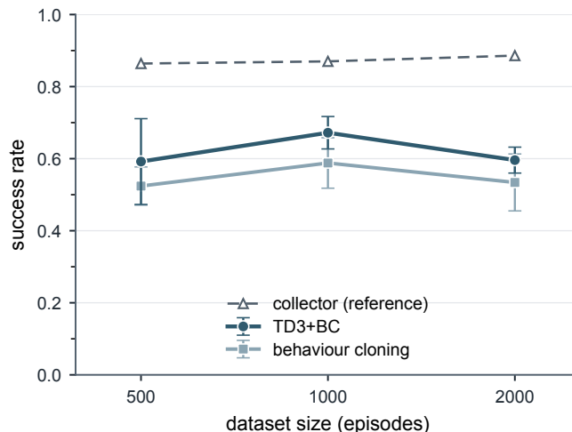
图 5.10: 亚临界横流穿越任务下可部署离线成功率随数据规模的变化（横流补偿参照采集、历史效率导向奖励、 s_0 单点传感、 k = 4 历史堆叠，正式五随机种子、终检评估）。TD3+BC（深色圆点）与同预算纯行为克隆（浅色方点）均在一千回合处达到峰值、在两千回合处回落，误差棒为跨随机种子标准差；灰色虚线为采集器自身轨迹的成功率，随规模反而轻微上升。数据越多、且采集轨迹越干净，可部署策略却越差，指向数据支持集的结构而非样本数量或数据质量。
