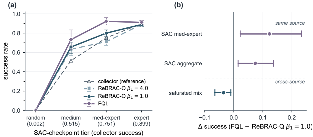
图 5.15: 算法与数据质量的交互（本章算法比较的核心图）。(a) SAC 检查点四档质量阶梯（横轴括号内为采集器自身成功率）上三个固定配置的终检成功率（三种子均值，误差棒为跨种子标准差；灰色虚线为采集器参考水平）：FQL 恰在非饱和的中段质量区间拉开优势（中等偏专家档 0.922 对 0.800），随机档三者皆零、专家档三者同收敛于采集器水平附近。(b) FQL 与 ReBRAC-Q \beta_1=1.0 之差及其 95% 配对自助置信区间：同源的 SAC 中等偏专家档 (+0.123) 与三档聚合 (+0.074) 严格为正，跨源补充的饱和混合单元 (-0.035) 严格为负——方向随数据质量区间翻转，且两侧区间均不含零。虚线分隔的跨源一侧使用不同的数据集与评估协议，仅支撑方向读数，两侧幅度不可直接比较。
