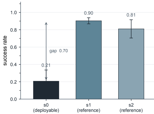
图 5.5: 临界工况 ( Re = 250 、 U_{\infty} = 1.5 m/s, 到达导向奖励) 下三种传感配置的任务成功率 (均值 \pm 标准差)。可部署单点 s_0 几近失败, 仅增设一处前向探针的 s_1 即守住约 0.90, 信息更丰富的 s_2 居中且离散度更大; 可部署配置与空间参照之间张开约 70 个百分点。 s_1 、 s_2 为参照上界, 在部署中不可得。该临界传感筛查为云端新近完成的初步结果 (PRELIMINARY), 逐次训练日志尚未取回本地核对 (见 §5.5.6)。
