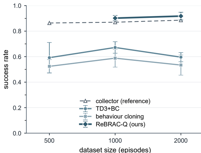
图 5.11: 横流补偿参照数据上可部署离线成功率随数据规模的变化: 双侧行为约束对回落的翻转 (历史效率导向奖励、亚临界工况、 s_0 单点传感、 k = 4 历史堆叠; 正式五随机种子协议、终检评估, 误差棒为跨随机种子标准差)。TD3+BC (圆点) 与同预算纯行为克隆 (方点) 两条序列与图 5.10 同源, 均在一千回合处最高、两千回合处回落; ReBRAC-Q (菱形, 双侧行为约束) 保持在采集成功率参照 (灰色虚线) 以上的水平, 两千回合不再低于一千回合。ReBRAC-Q 未在五百回合数据上训练, 其序列自一千回合起; 其两千与一千回合两点的差异未作显著性检验, 只读作回落不再出现 (正文)。
