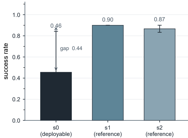
图 5.5: 临界工况 ( Re = 250 、 U_\infty = 1.5 m/s, 到达导向奖励) 下三种传感配置的任务成功率 (均值 \pm 标准差)。可部署单点 s_0 在重复训练间剧烈分化、均值仅约 0.46, 仅增设一处前向探针的 s_1 即一致守住约 0.90, 信息更丰富的 s_2 与 s_1 几乎并列; 可部署配置与空间参照之间张开约 44 个百分点。 s_1 、 s_2 为参照上界, 在部署中不可得。
