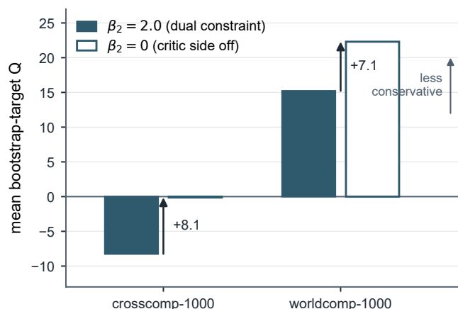
图 5.12: 移除价值侧支持惩罚 ( \beta_2 = 0 ) 后自举目标 Q 的跨数据集同向漂移。纵轴为训练后期窗口内的平均自举目标 (诊断量, 读取自价值侧惩罚施加之前, §5.7.6)。横流补偿参照数据 (图中 crosscomp-1000) 与世界坐标系流速补偿参照数据 (图中 worldcomp-1000) 的完整配置基线 (实心柱) 位于零的两侧, 移除该惩罚 (空心柱) 后二者都朝更不保守的方向漂移 +7 至 +8 个绝对单位 (箭头), 相对幅度分别约 +98% 与 +46%。横流补偿参照数据的消融为五随机种子, 世界坐标系流速补偿参照数据的为两随机种子探查。
