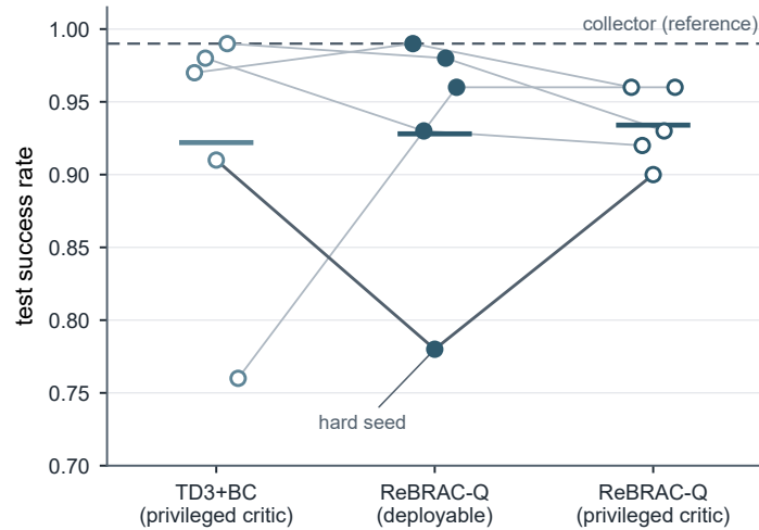
图 5.11: 世界坐标系流速补偿参照数据（亚临界工况、历史效率导向奖励、 s_0 单点传感、 k = 4 历史堆叠）上三种协议的种子级终检成功率（五随机种子、每种子 100 回合；纵轴自 0.70 起；细线连接同一随机种子，短横杠为各协议均值，虚线为采集器自身成功率 0.990 的参照水平；实心点为可部署协议，空心点为特权协议）。可部署协议下的 ReBRAC-Q（中列）与训练期接收特权观测的 TD3+BC（左列）处于同一水平，二者未检测到统计显著差异（正文）；把特权协议施加到 ReBRAC-Q 自身（右列）几乎不改变均值，其作用集中于把可部署协议下唯一的难例种子（深色连线，图中标注 hard seed）由 0.780 救回 0.900，其余种子保持原位或轻微下移。
