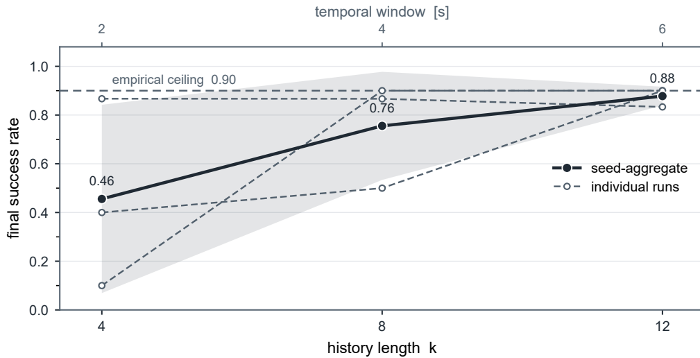
图 5.8: 临界工况下可部署单点 s_0 的最终成功率与其跨重复训练离散度随观测历史长度 k 的变化 (终检评估; 上轴为对应时序窗 k \cdot \Delta t_{\text{ctrl}} , \Delta t_{\text{ctrl}} = 0.5 \text{ s} )。深色为三次重复训练的聚合趋势 (均值与种子带), 浅色细线为三次训练各自的轨迹: 两次沿 k = 4 \rightarrow 8 \rightarrow 12 未见回落, 一次在高位持平后微降。判别力来自同一初始化下的跨历史长度对照, 即 k = 8 时停在中途的那次训练在仅改变历史长度后被推到经验上界 (0.90, 灰色虚线); 离散度随 k 的收窄与之一致, 只作旁证。
