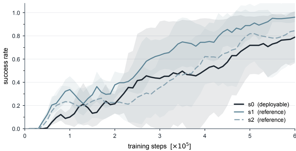
图 5.4: 亚临界主工况 ( Re = 150 、 U_\infty = 1.0 m/s, 历史效率导向奖励) 下三种传感配置的在线学习曲线, 以标准 SAC 训练、确定性策略评估所得任务成功率 (均值与种子带, 曲线经轻度滑动平均)。三种配置均可学; 信息最丰富的 s_2 训练过程的离散度全程大于 s_1 , 更多观测通道未换来更稳的训练。 s_1 、 s_2 为参照上界, 在部署中不可得。
