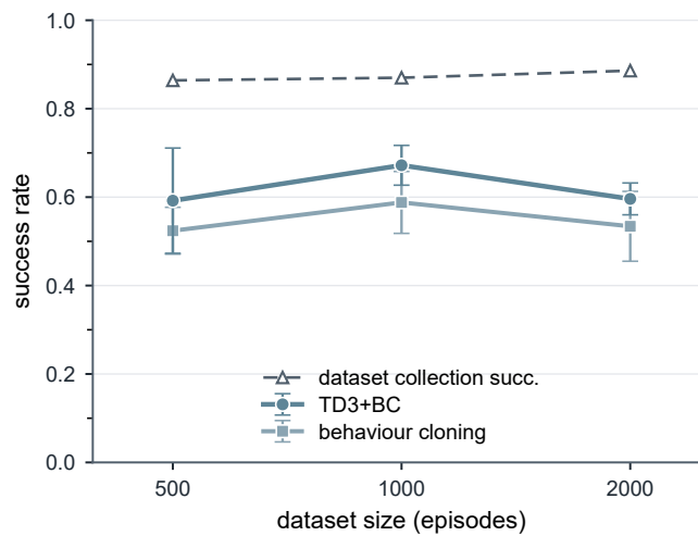
图 5.10: 亚临界横流穿越任务下可部署离线成功率随数据规模的变化（横流补偿参照采集、历史效率导向奖励、 s_0 单点传感、 k = 4 历史堆叠，正式五随机种子、终检评估）。TD3+BC（深色圆点）与同预算纯行为克隆（浅色方点）均在一千回合处最高、在两千回合处回落，误差棒为跨随机种子标准差；灰色虚线为采集器自身轨迹在采集回合上的成功比例，即数据集采集成功率，随规模反而轻微上升。数据越多、且采集轨迹越干净，可部署策略却越差，指向数据支持集的结构而非样本数量或数据质量。
