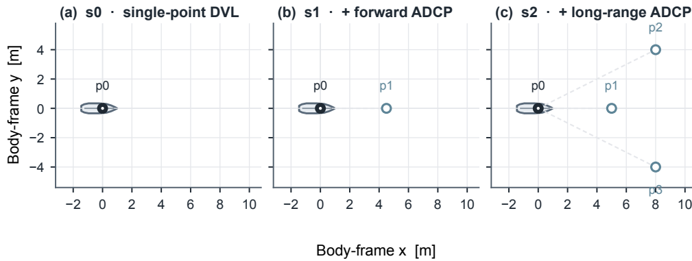
图 5.1: 本章三种传感配置的体坐标系探针几何。(a) s_0 仅在机体质心设单一 DVL 水追踪探针，是可部署主轴；(b) s_1 在 s_0 之外增设一处前向探针（机体前方 4.5 m），对应短程前视 ADCP，提供约三个控制步的轴向预警；(c) s_2 进一步增设近端前向（5 m）与两侧（纵向 8 m、横向 \pm 4 m）探针，对应长程前视 ADCP，兼具约七步的轴向预警与侧向流速梯度。实心圆为质心单点探针，空心圆为增设的前向 / 侧向探针； s_1 与 s_2 仅作参考上界。
