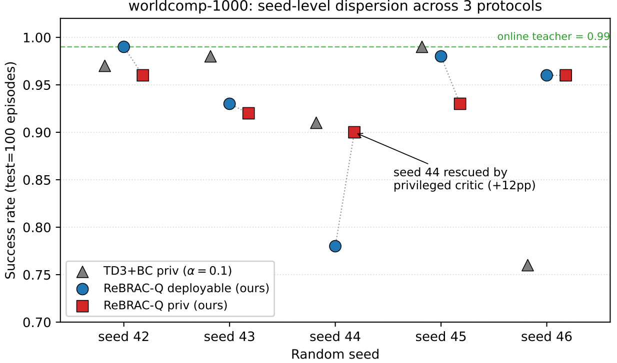
图 1: seed-level success rate 分布 (worldcomp-1000, test=100 episodes) 。横轴为 5 个 random seeds (42–46)，纵轴为成功率。三种协议：(i) TD3+BC privileged-critic ( \alpha = 0.1 , 灰色三角)；(ii) ReBRAC-Q deployable-only (蓝色圆点)；(iii) ReBRAC-Q privileged-critic (红色方块)。同一 seed 之间用细虚线连接，便于读出“deployable→privileged”在 seed 内部的位移。 关键观察 ：seed 44 在 ReBRAC-Q deployable-only 下显著低于其他 seed (0.78 vs 0.93–0.99)，切换到 privileged-critic 后被救回到 0.90 (+12pp)；其他 seed 的“deployable→privileged”位移均在 \pm 3\text{pp} 内，方向并不一致——privileged-critic 在 ReBRAC-Q 上的 mean 抬升完全由 seed 44 这一个 outlier 提供。
