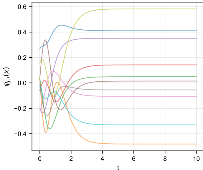
RA-PIKAN — Layer 2
