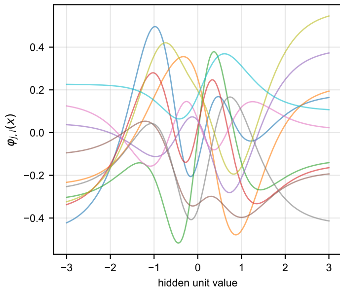
RA-PIKAN — Layer 2
