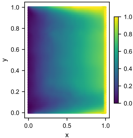
RA-PIKAN (ours)
