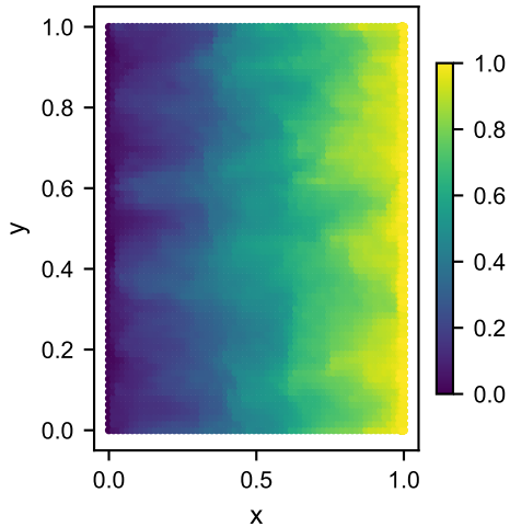
RA-PIKAN (ours)
