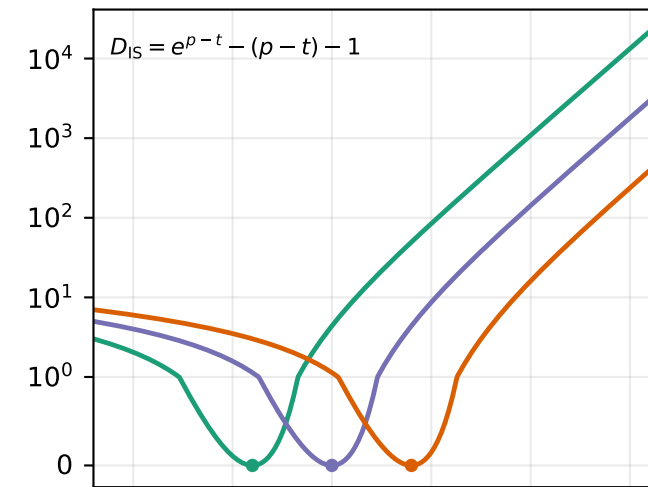
Itakura-Saito
