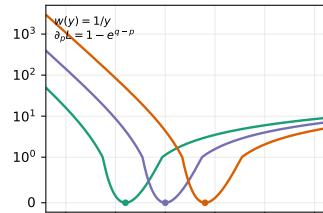
Itakura--Saito
