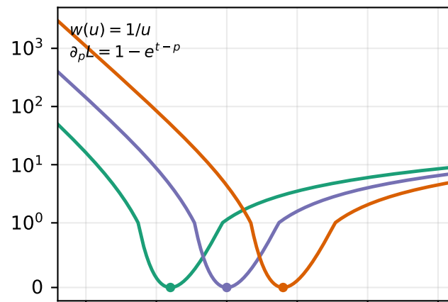
Itakura--Saito
