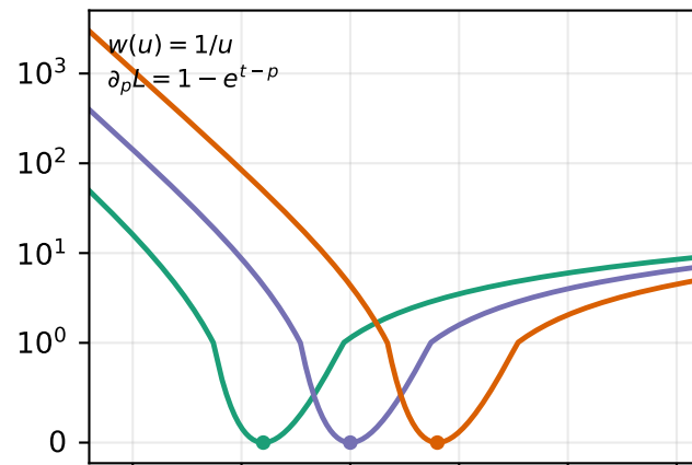
Itakura--Saito
