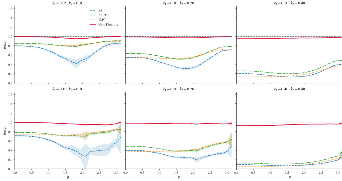
展示了共 16 个模拟实现与 N 体模拟在不同构型下的双谱比值，横轴为两波矢夹角 \theta 。红色实线的新流程在各构型中更接近 1，而微扰论基准在非线形尺度上的双谱幅度偏低。
