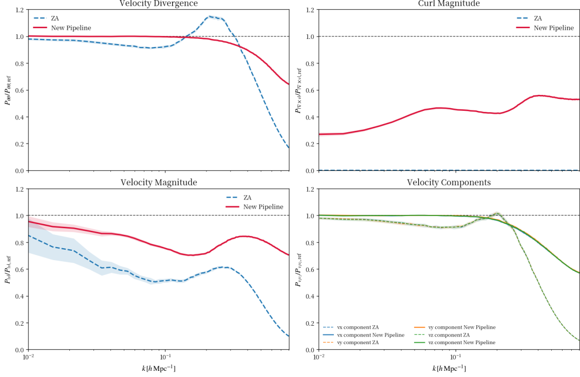
第 32–47 个模拟实现的速度场功率谱以 N 体模拟为参考。左上：速度散度功率谱比值 P_{\theta\theta}/P_{\theta\theta,\text{ref}} ；右上：速度旋度模功率谱比值 P_{|\nabla \times v|}/P_{|\nabla \times v|,\text{ref}} ；左下：速度模功率谱比值 P_v/P_{v,\text{ref}} ；右下：三个速度分量功率谱比值 P_{v_i}/P_{v_i,\text{ref}} 。虚线为 ZA，实线为新流程，阴影为不同实现的 1\sigma 散布。
