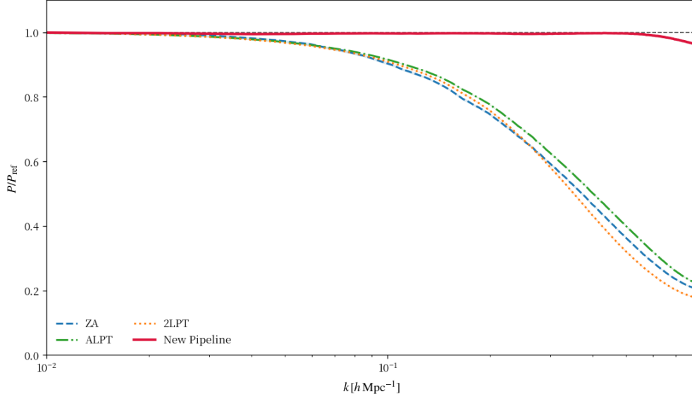
展示了 16 个模拟实现与 N 体模拟的功率谱比值，曲线为不同实现的均值，阴影为 1\sigma 散布，散布很小；ZA、2LPT 和 ALPT 在小尺度逐渐低估功率，而新流程在接近 Nyquist 波数前整体保持在 1 附近。
