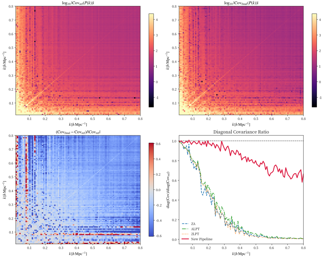
协方差矩阵由 48 个模拟实现估计得到，采用线性 k 分箱。左上：N 体参考功率谱协方差矩阵的 \log_{10} |\text{Cov}_{\text{ref}}(P(k))| ；右上：新流程功率谱协方差矩阵的 \log_{10} |\text{Cov}_{\text{final}}(P(k))| ；左下：新流程相对 N 体参考协方差矩阵的逐元相对差异；右下：ZA、ALPT、2LPT 和新流程的协方差对角元相对 N 体参考的比值。
