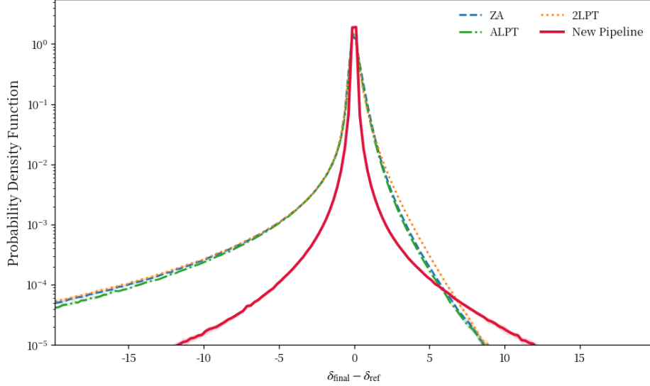
曲线统计了 16 个模拟实现与 N 体模拟的过密度残差的概率密度分布，阴影表示不同实现的 1\sigma 散布，散布很小；ZA、2LPT 和 ALPT 的残差分布尾部更宽，新流程的残差更集中于 0 附近，说明单点统计恢复更接近 N 体结果。
