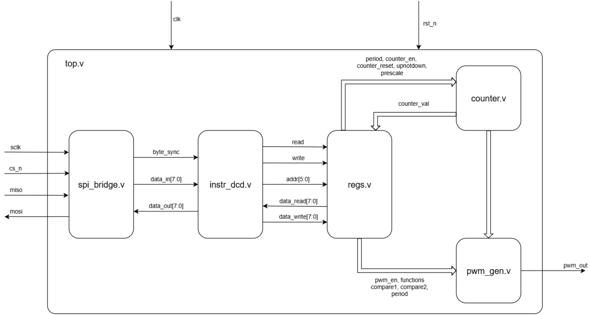
Figure 1: Schema bloc a generatorului de semnal PWM
