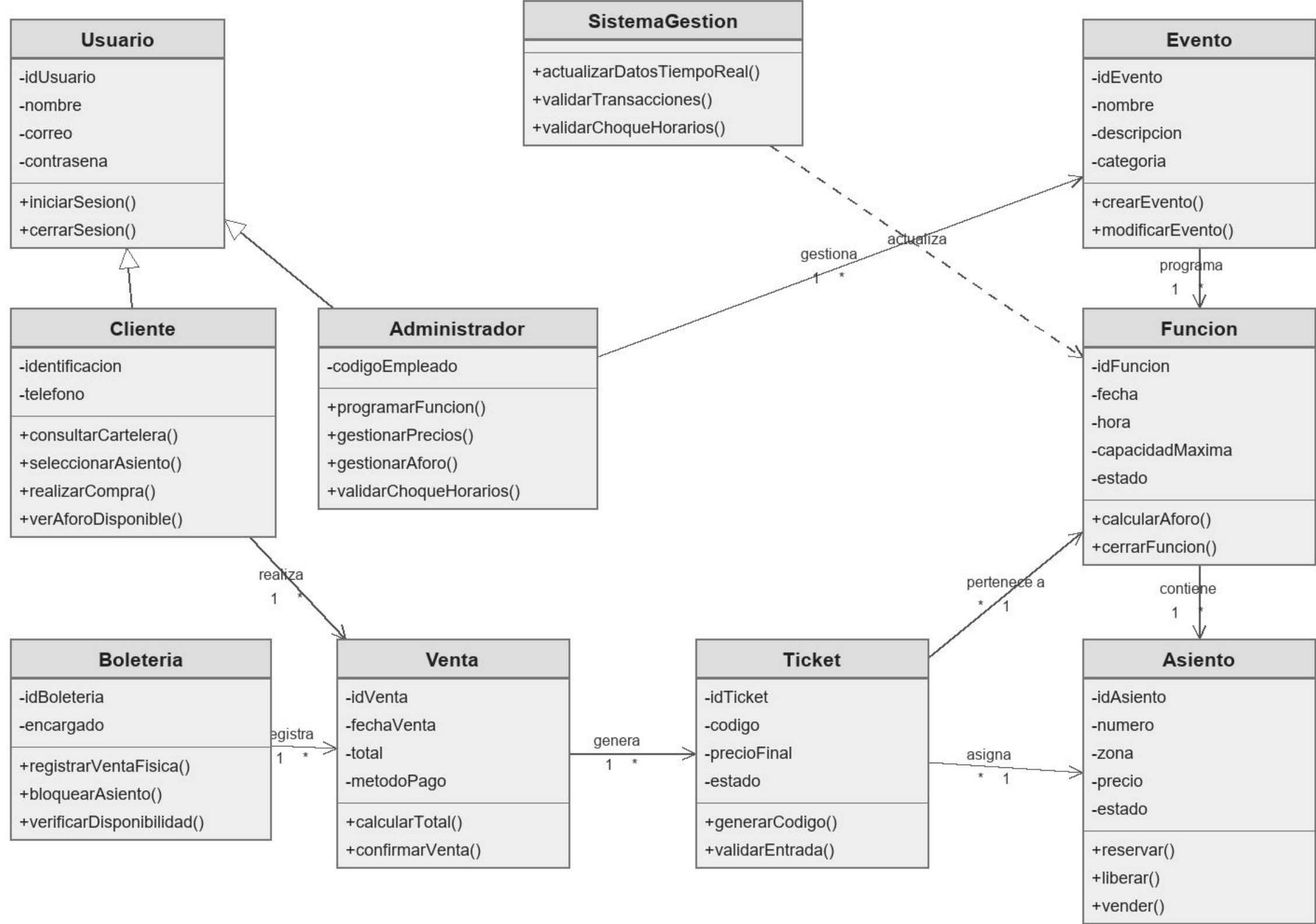
Diagrama UML de Clases - Sistema de Circo
