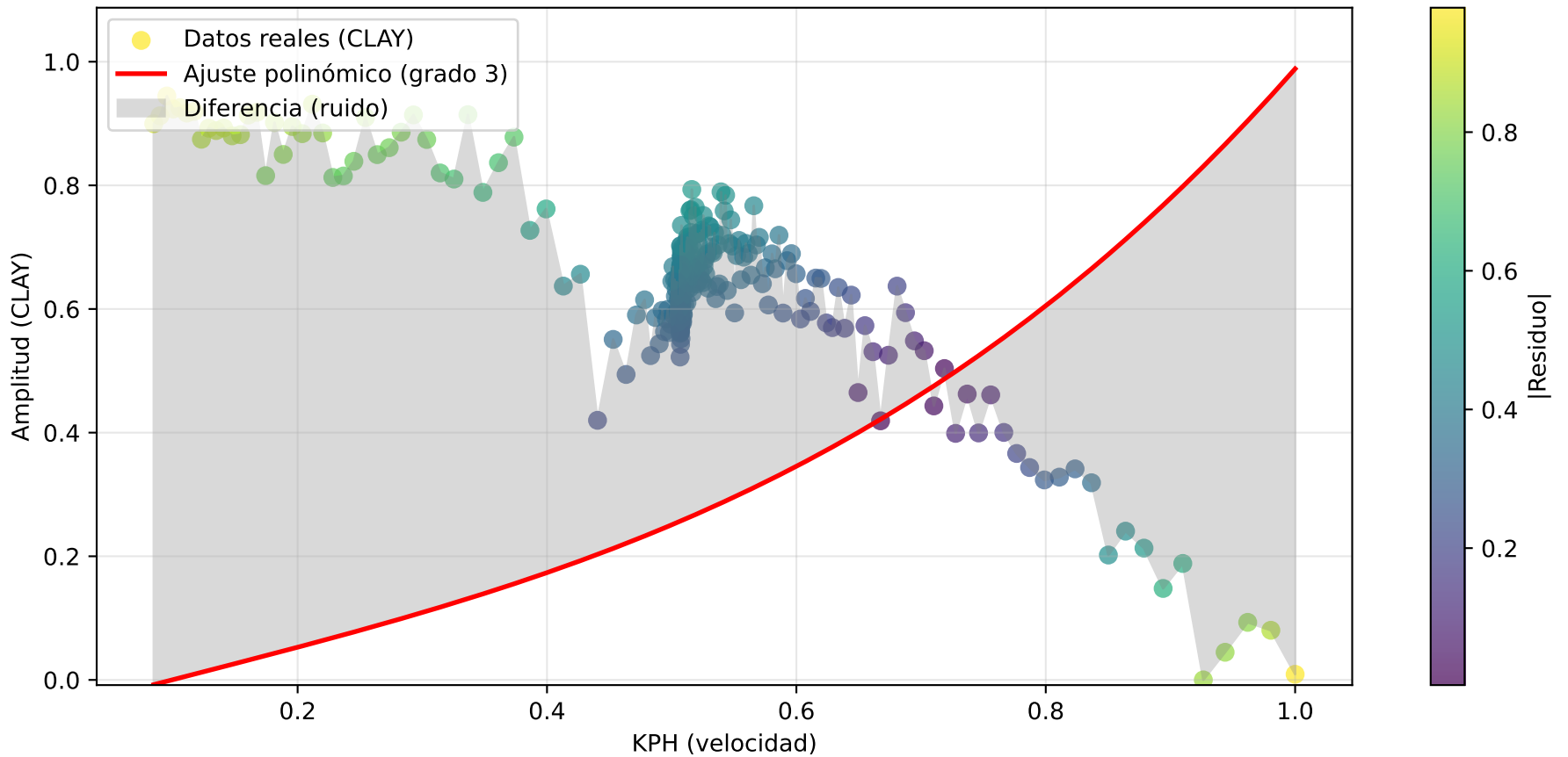
CLAY - P(Desalineación) = 0.9128
