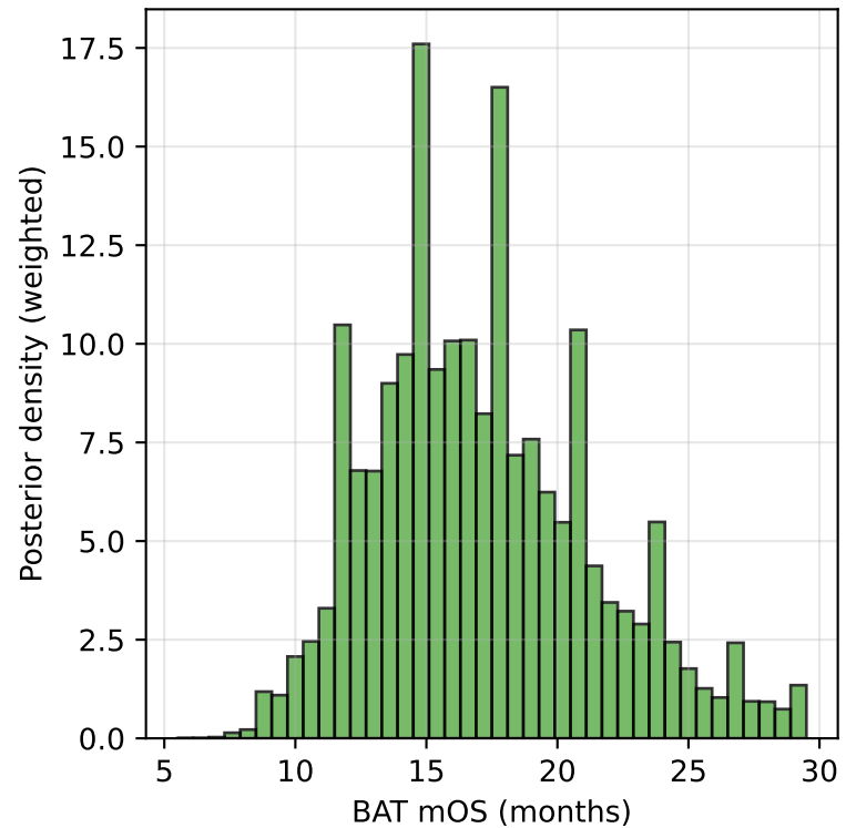
BAT mOS posterior (no biological prior)
